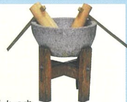
●もちつき (本体φ500・H210mm) (石うす台 H485mm) ※キネ別途
